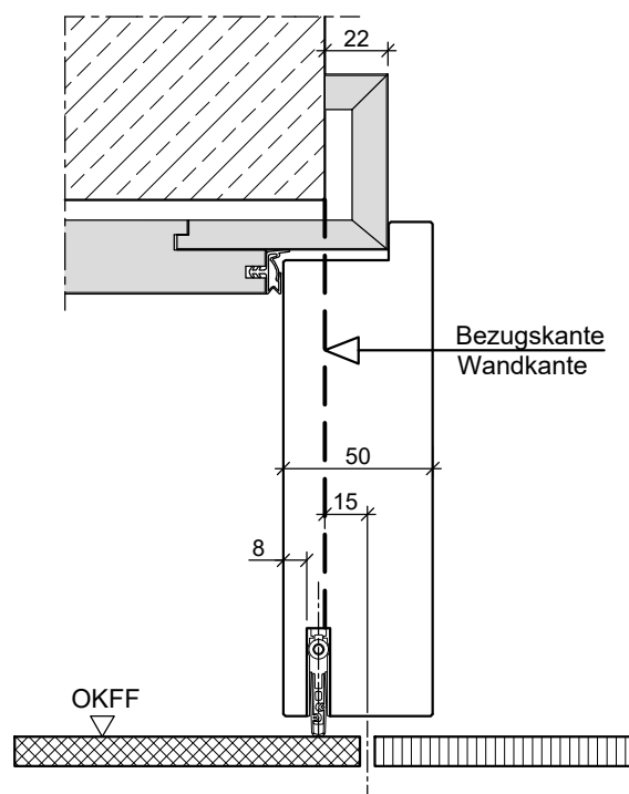
HW50-gefalzt in Holzumfassungszarge
