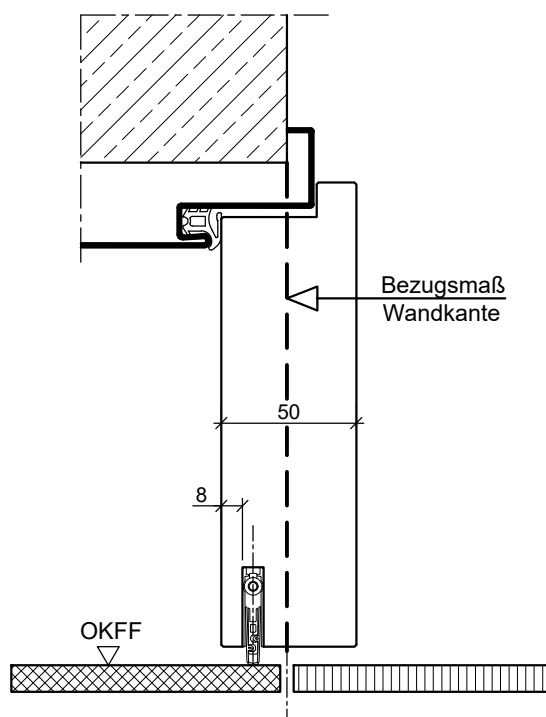
HW50-gefalzt Stahlzarge
